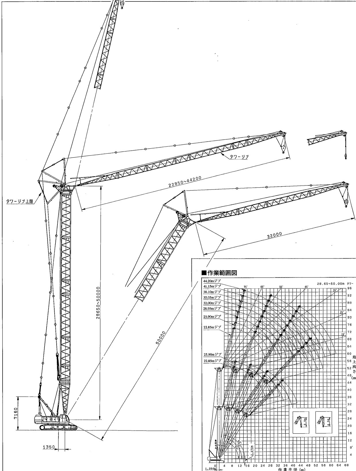
■基本寸法図
