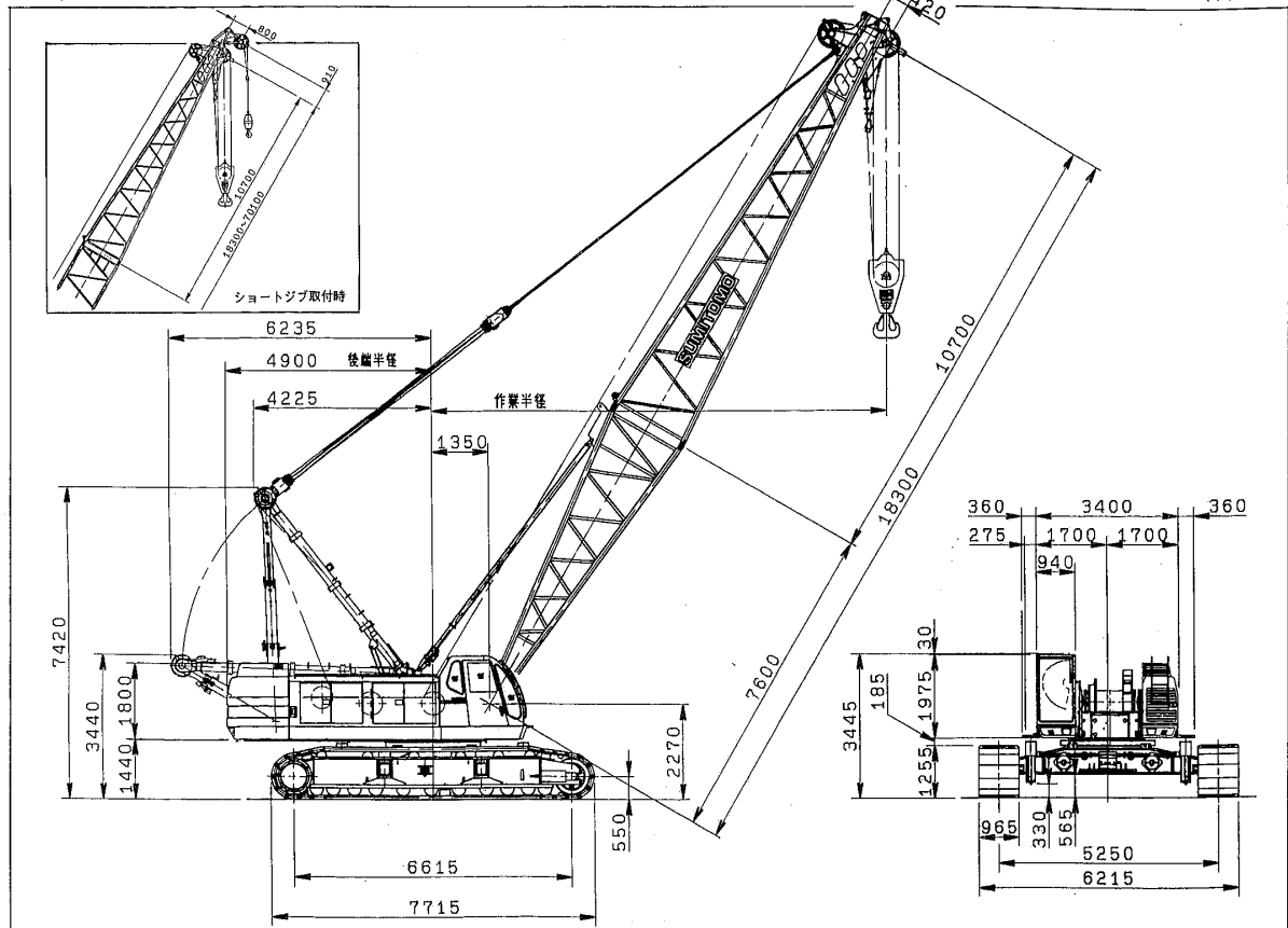
■基本寸法図
