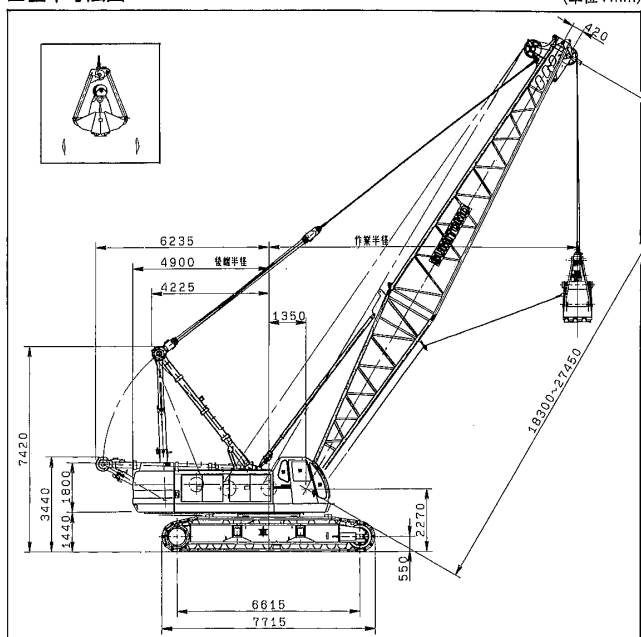
■基本寸法図
