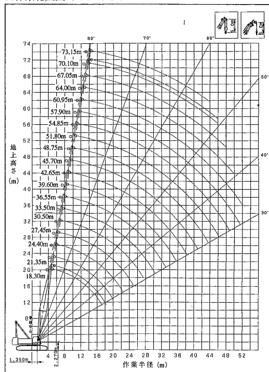
■作業範囲図 クローラクレーン
